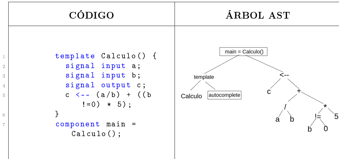
Figura 4.1: Construcción de AST
